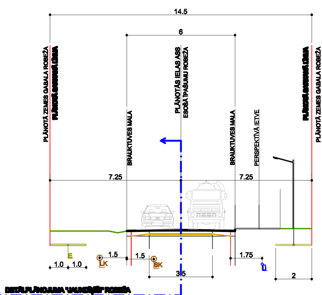
ŠKĒRSPROFILS A-A
