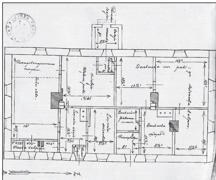
Suntažu pagasta nama plāns 1924.gadā. (LVVA 3723.fonds, 1.apraksts, 16309.lieta, 131.lp.)
