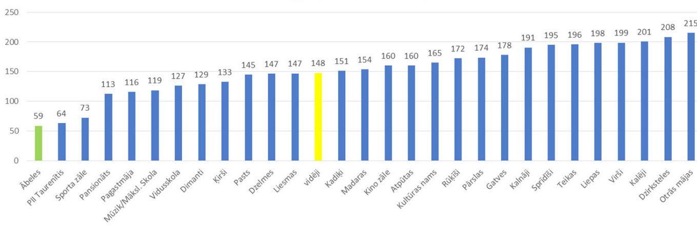
Enerģijas patēriņš kWh/m 2 gadā
