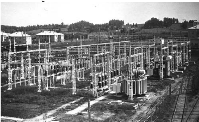
88 kV sadales būve 1939.g. vasarā
